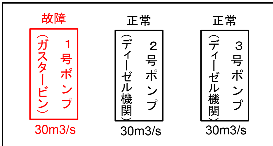
久御山排水機場ポンプ配置図
